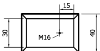
Fundamentsockel R Art-Nr.: 15-4006-XXR-0-000 Hülse M16 Gewicht: 84 kg
